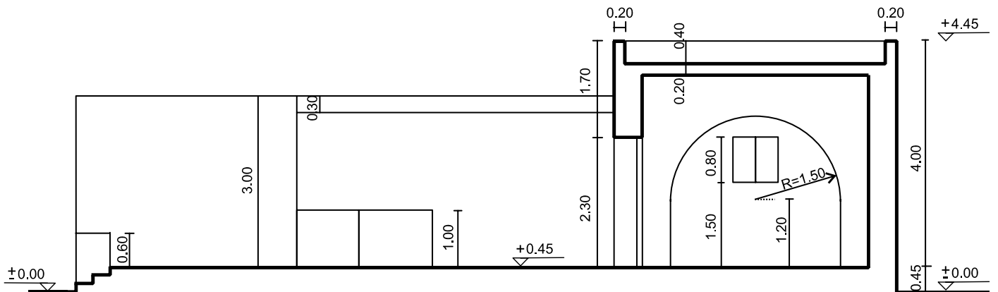
ΤΟΜΗ Α-Α
